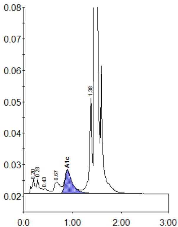
Peak table - ID: 10412780
